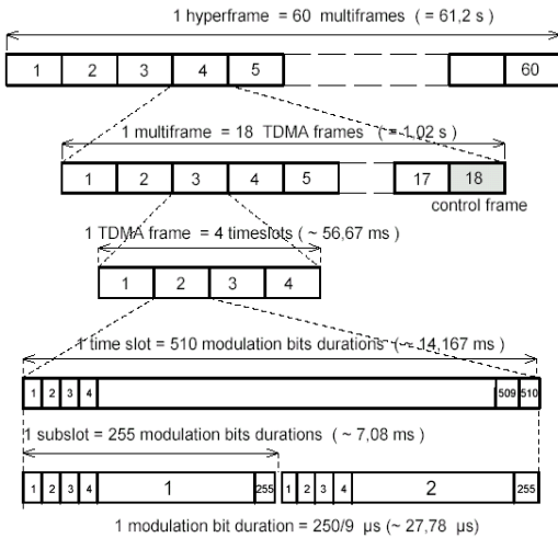
Fig. 3. Formatação dos quadros de dados TDMA/Tetra
