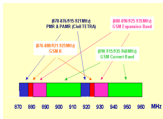
Fig. 2. Distribuição de canais do Tetra na Europa
