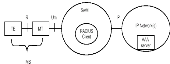
Fig.4. Autenticação da estação Tetra
