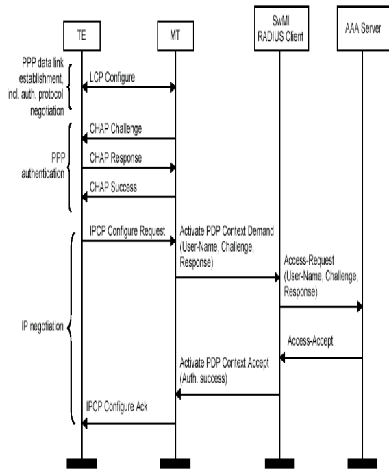
Fig. 5. Negociação de protocolos para conexão Tetra Fonte: Adaptado de ETSI EN 300.392-2, v.2.5.2/2005
