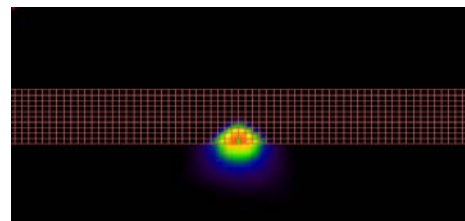
Fig. 6 – Representação da Intensidade instantânea da energia eletromagnética atravessando uma estrutura.
