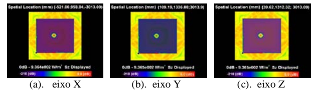
Fig. 5 – Componentes Z do vetor de Poynting ( S_z ), considerando a maior anisotropia.
