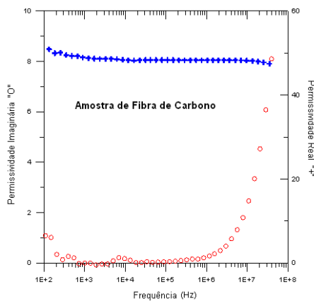
Figura 3 – Medida de permissividade complexa do CFC.
