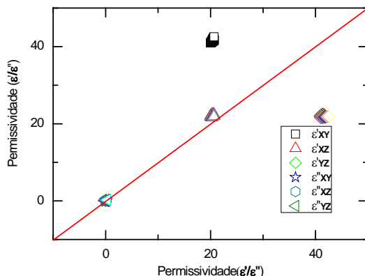
Fig. 4. Dados de permissividades, partes real e imaginária, confrontando-se em relação dos eixos
