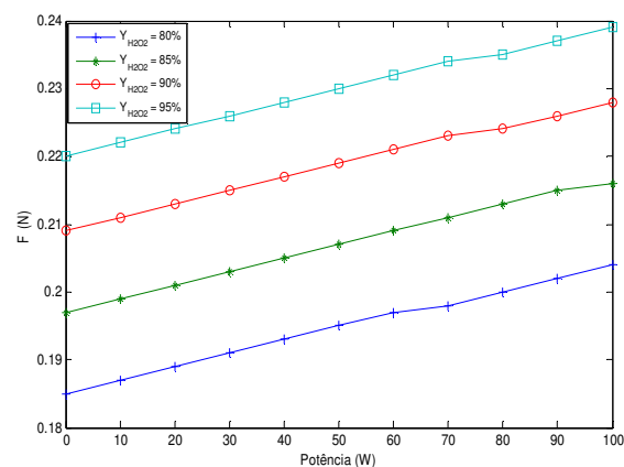
Fig. 4. Empuxo versus potência elétrica fornecida.
