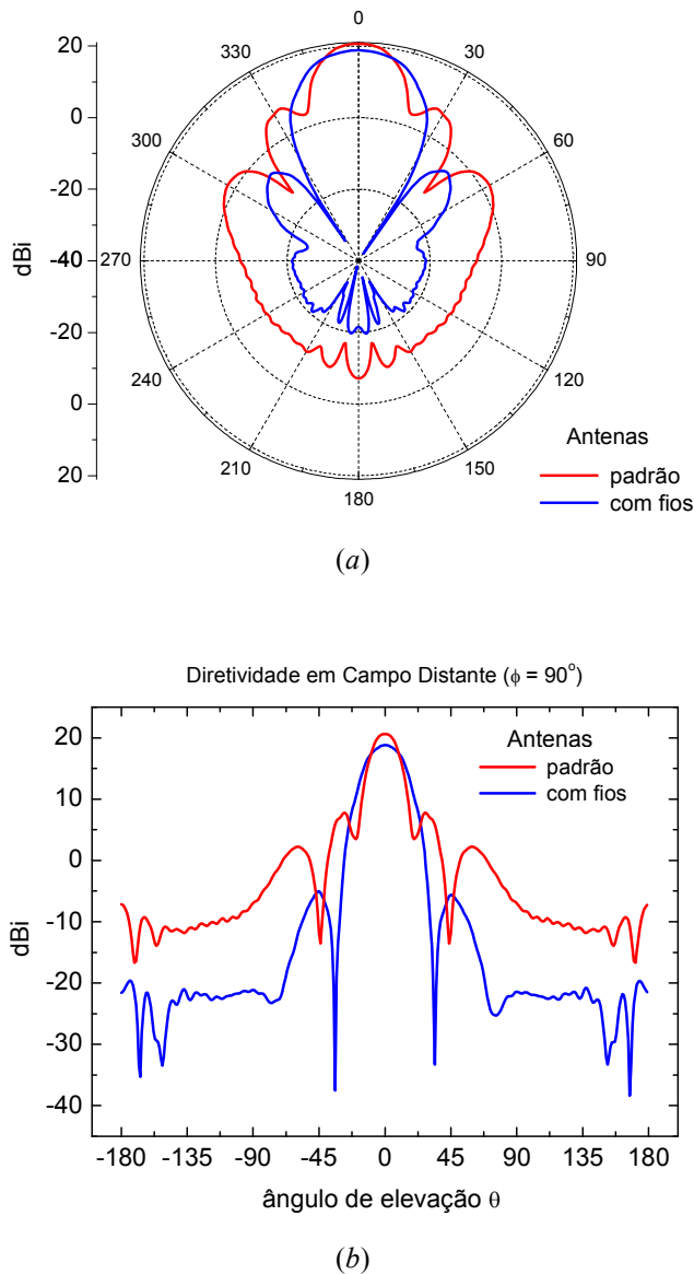
Fig.8. Diretividade da antenna convencional padrão e da antenna carregada com fios condutores metálicos na forma polar (a) e cartesiana (b) na frequência de 9,5 GHz.
