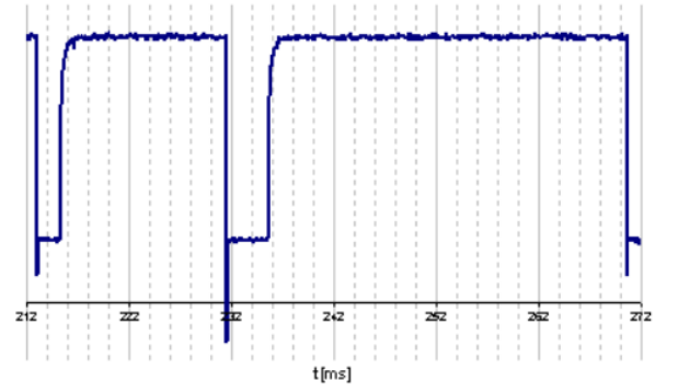
Fig. 3: Forma de onda de saída real do sensor.
