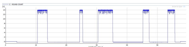
Fig. 15: Forma de onda do Sensor B1 (5 rajadas).
