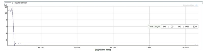
Fig. 10: Largura de pulso (1.3 ms).
