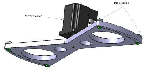
Fig. 4: Alvos instalados nas pás.
