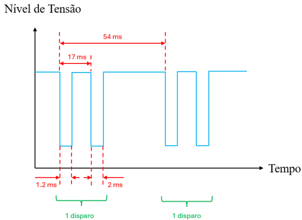
Fig. 2: Forma de onda de saída teórica do sensor.
