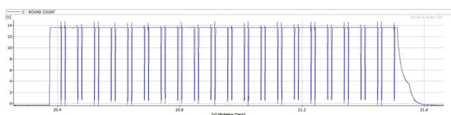
Fig. 14: Forma de onda do Sensor A1 (Rajada #2).
