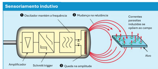
Fig. 1: Topologia típica de um sensor indutivo de proximidade.
