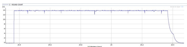
Fig. 16: Forma de onda do Sensor B1 (Rajada #2).
