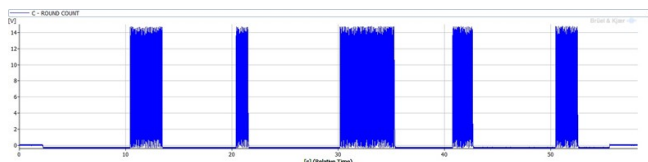
Fig. 13: Forma de onda do Sensor A1 (5 rajadas).
