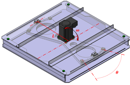
Fig. 6: Principais parâmetros do dispositivo de teste.
