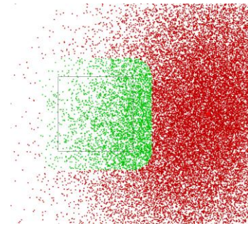
Fig. 8 – Simulação Monte Carlo dos pontos de impacto de lançamento de armamento em rastilho interagindo com uma CDRO
