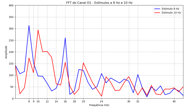
Fig. 4: Espectro de frequência dos sinais EEG após FFT para estímulos de 8 Hz (azul) e 10 Hz (vermelho).
