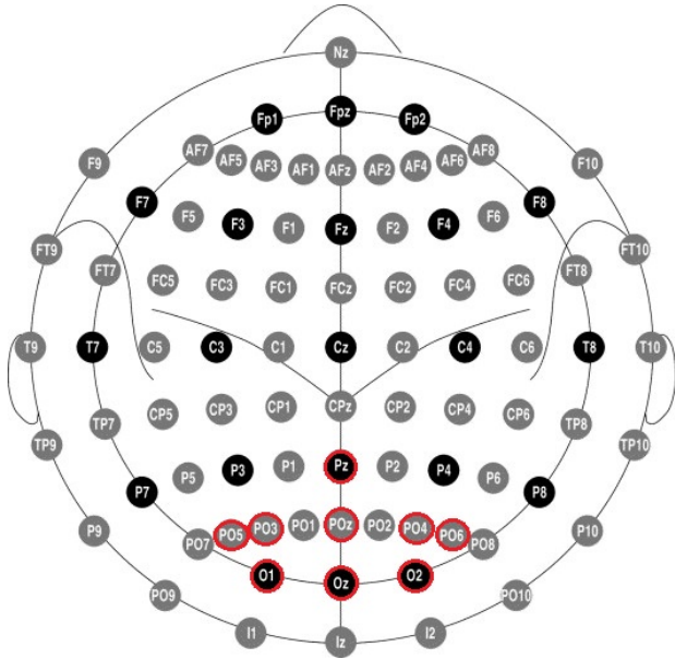
Fig. 3: Distribuição dos eletrodos no escalpo conforme o sistema internacional 10-10. As nove posições destacadas em vermelho correspondem aos canais seleccionados nas regiões occipital, parietal e parieto-occipital, que apresentam relevância para a detecção de SSVEP. (Figura adaptada de [12]).
