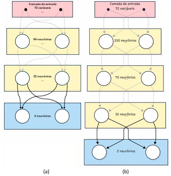
Fig. 5: Arquitetura dos classificadores. (a) Modelo da MLP do Cenário 1. (b) Modelo da MLP dos Cenário 2 e 3.
