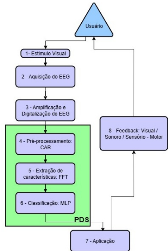
Fig. 1: Diagrama das etapas de um sistema BCI-baseado em SSVEP.
