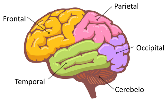
Fig. 2: Representação esquemática dos principais lobos do cérebro humano. É na região do lobo occipital onde os sinais SSVEP são primariamente gerados em resposta a estímulos visuais intermitentes.
