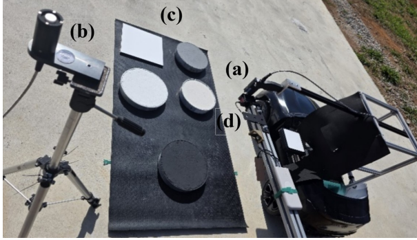
Fig. 3. Arranjo experimental para as metodologias de caracterização radiométrica em campo, com (a) um FieldSpec para medição de radiância, e (b) um FieldSpec para medição de irradiância, (c) superfícies refletoras (Spectralon; branca; cinza claro; cinza escuro; e preta), e (d) câmera Parrot Sequoia fixada ao nadir das superfícies.
