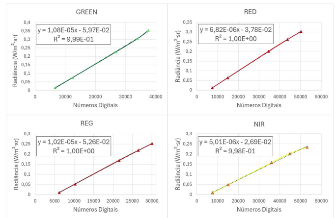
Fig. 9. Curvas de caracterização radiométrica, por sensor, para a metodologia por variação de superfície.
