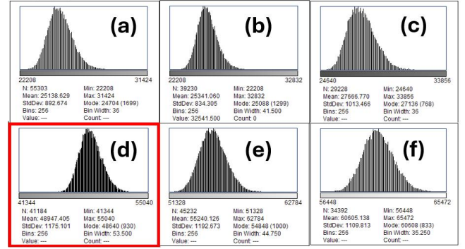
Fig. 4. Sequência de histogramas dos números digitais das imagens coletadas referentes ao 1º turno de medições, para o sensor NIR. ISO mantido em 100, e Exp Time (em \mu s) variando de (a) a (f), conforme Tabela II.
