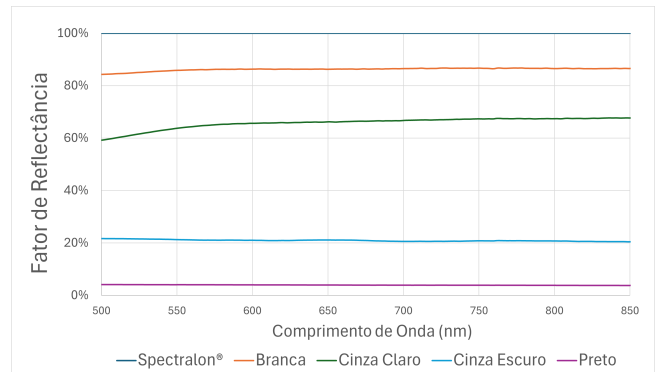
Fig. 5. Fatores de Reflectância das superfícies utilizadas.
