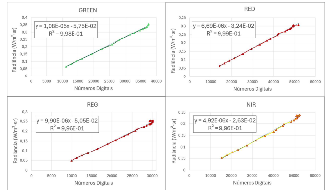
Fig. 8. Curvas de caracterização radiométrica, por sensor, para a metodologia por variação da irradiância solar.
