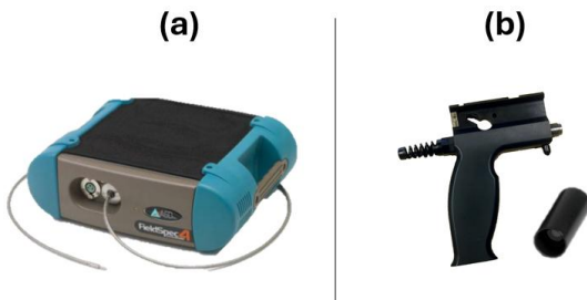
Fig. 1. Espectrorradiômetro de Campo (a) FieldSpec 4, com guia de fibras ópticas acopladas a um (b) suporte de fibra e limitador de FOV de 8°.
