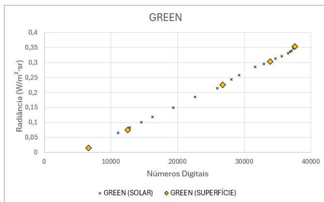
Fig. 10. Pontos das retas de caracterização radiométrica por variação solar e de superfície, sobrepostos, para o sensor Green .
