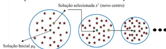
Fig. 1. Ideia geral da rotina de busca do VS, traduzida de [3].
