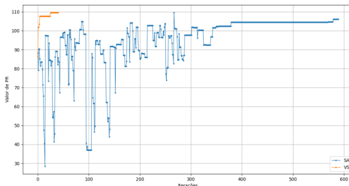
Fig. 2. Gráfico de convergência comparativo entre o VS e o SA.
