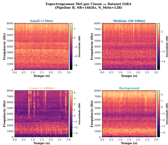
Fig. 1. Espectrogramas Mel das quatro classes do dataset IARA, apresentados com escala de intensidade comum (percentis 2–98) para permitir comparação visual direta. Small (<50 m): linhas tonais esparsas de banda estreita; Medium (50–100 m) e Large (>100 m): harmônicos densos com energia crescente em baixas frequências; Background : ruído oceânico estocástico de baixa frequência (DC E). Eixo X: tempo (s); Eixo Y: frequência (Hz).
