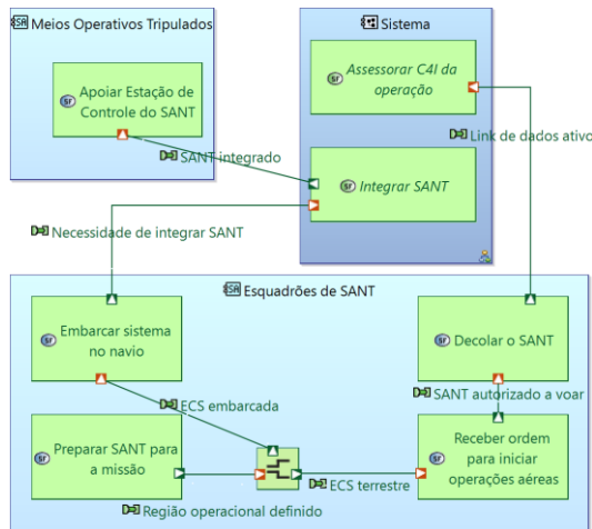
Fig. 3. Extrato do Diagrama de Análise de Sistemas (SAB).
