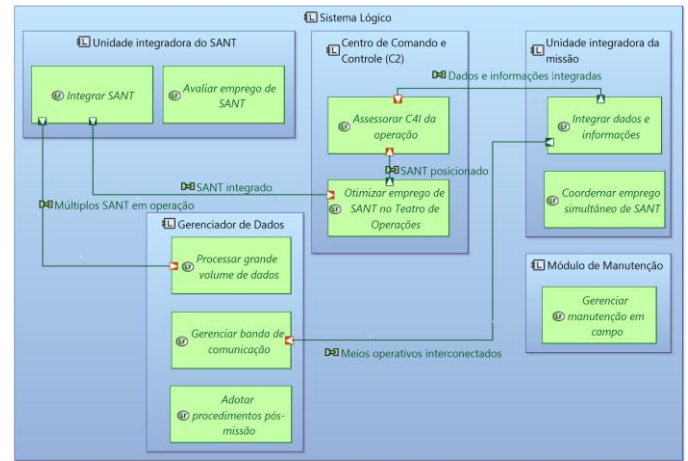
Fig. 5. Extrato do Diagrama de Arquitetura Lógica (LAB).
