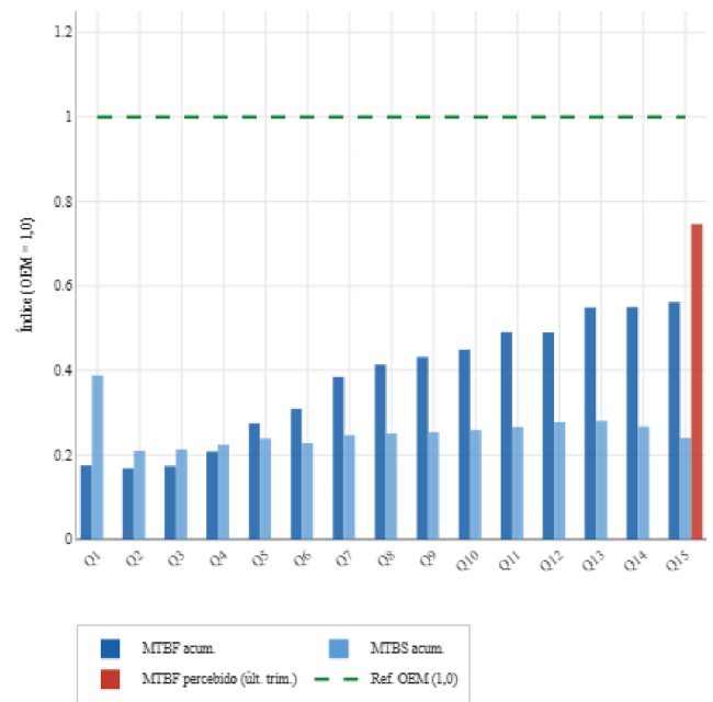
Fig. 1. Evolução do MTBUR e do MTBS da frota por trimestre, normalizados pelo OEM (índice = 1,0). No último trimestre, barra vermelha = MTBUR percebido pelos técnicos. Linha verde tracejada = referência OEM.
