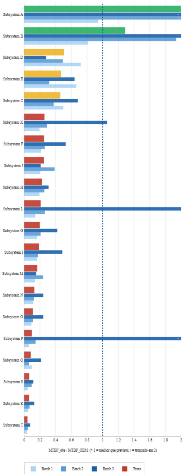
Fig. 3. Razão MTBF_{obs}/MTBF_{OEM} por subsistema, decomposta por lote de incorporação (Batch 1 a 3) e frota completa. Barra da frota mais larga, colorida por faixa: verde=razão \geq 0,9 ; amarelo= [0,4; 0,9) ; vermelho < 0,4 . Eixo truncado em 2; marcador “)” = razão superior ao limite. Ordenação pela razão da frota.
