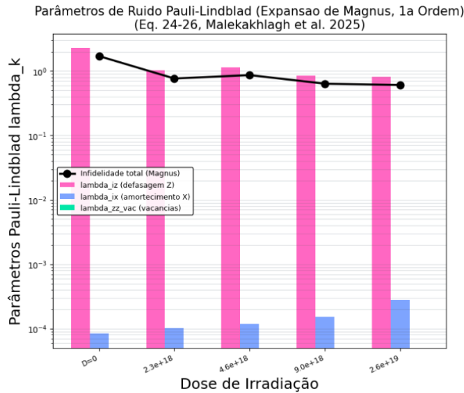
Fig. 4. Parâmetros de erro Pauli-Lindblad e infidelidade total obtidos via integração de Magnus de primeira ordem.
