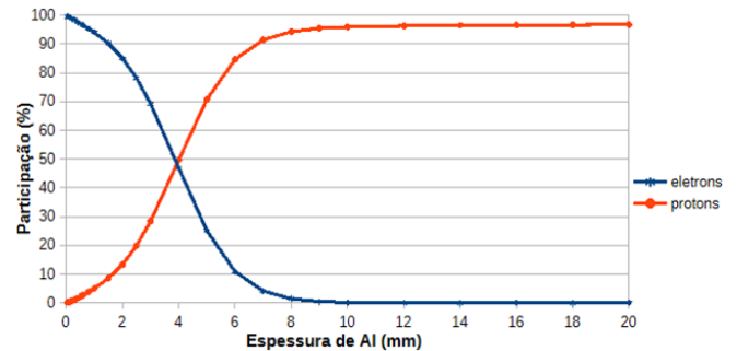
Fig. 4. Participação relativa dos elétrons e prótons aprisionados na Dose Ionizante Total em função da espessura da blindagem de alumínio.
