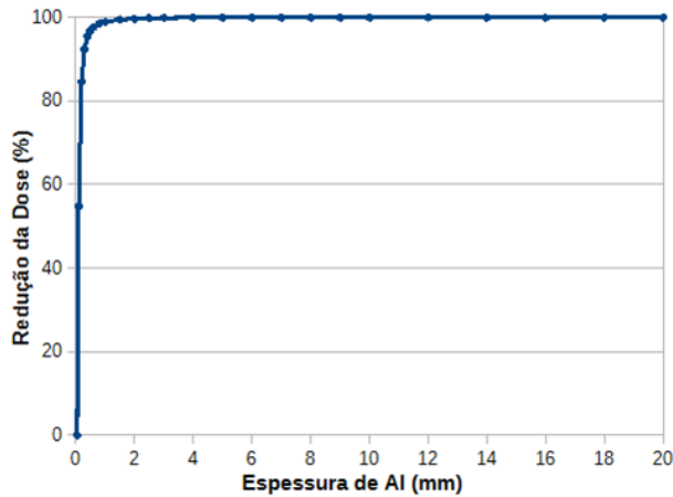
Fig. 2. Redução percentual da Dose Ionizante Total acumulada em relação à espessura de 0,05 mm.
