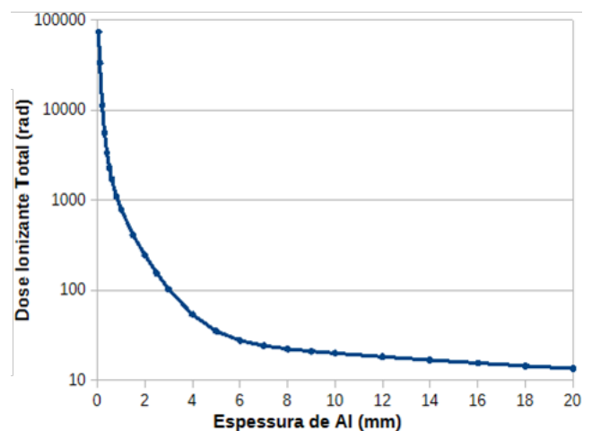
Fig. 1. Dose Ionizante Total acumulada em função da espessura de blindagem de alumínio.
