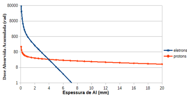
Fig. 3. Contribuição dos elétrons e prótons aprisionados para a Dose Absorvida acumulada.
