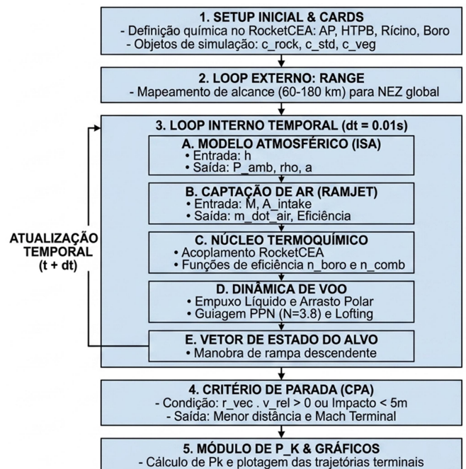
Fig. 3. Arquitetura do modelo de simulação
