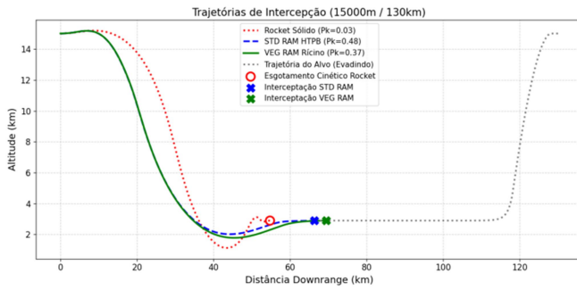
Fig. 4. Avaliação cinemática para a distância nominal de 130 km e 15 km de altitude inicial
