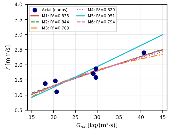
Fig. 2. Curvas ajustadas dos seis modelos sobrepostas aos dados do injetor axial ( N = 7 ).
