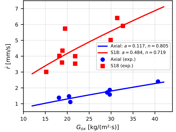
Fig. 1. Taxa de regressão versus fluxo de massa do oxidante para os injetores axial e S18, com lei de potência ajustada para cada configuração.
