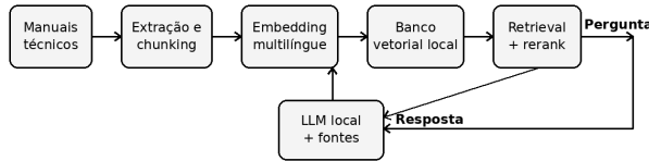
Fig. 1. Fluxo lógico do algoritmo RAG proposto. Fonte: elaboração própria.
