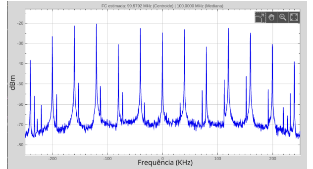
Fig. 8. Reconstrução do sinal PM ( \beta = 4,71 ) após ajuste do B_{lim} para 85 KHz, permitindo a unificação das raia dispersas.
