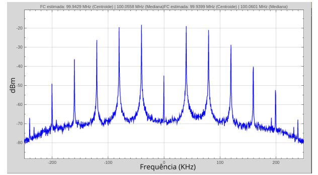
Fig. 7. Fragmentação do espectro para FM ( \beta = 2,4 ) com B_{lim} = 55 KHz.
