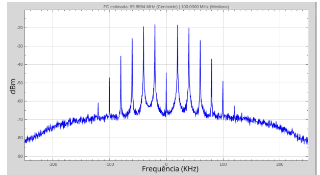
Fig. 4. Espectro capturado pelo RDS para o sinal FM com \beta = 2, 4 e f_m = 20 KHz.
