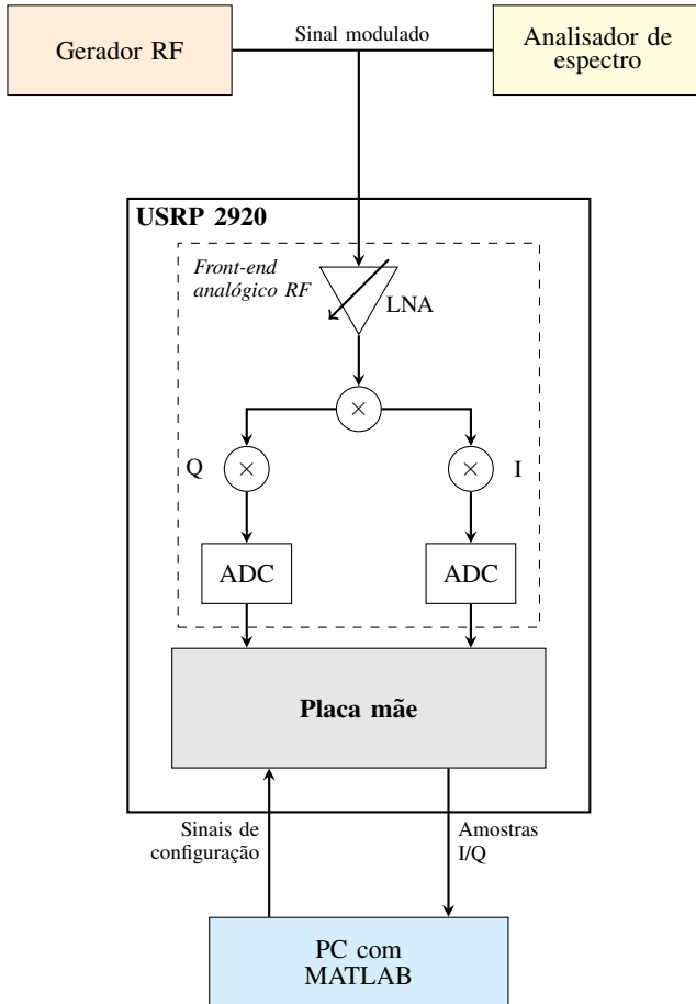
Fig. 2. Diagrama ilustrativo do setup experimental utilizado para captura dos sinais.
