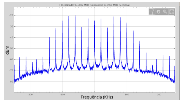
Fig. 5. Espectro capturado pelo RDS para o sinal PM com \beta = 4, 71 e f_m = 20 KHz.
