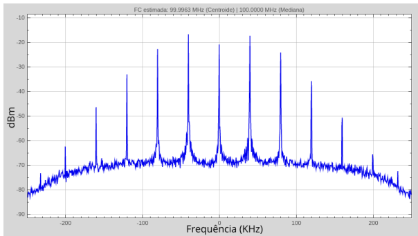
Fig. 6. Espectro capturado pelo RDS para o sinal FM com \beta = 1,7 e f_m = 40 KHz.
