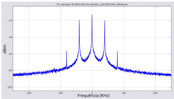
Fig. 3. Espectro capturado pelo RDS para o sinal AM com 100% de modulação e f_m = 40 KHz.
