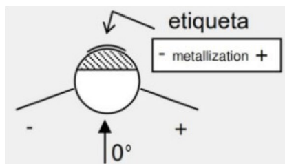
Fig. 3. Posição do refletor de Luneberg em relação as antenas.
