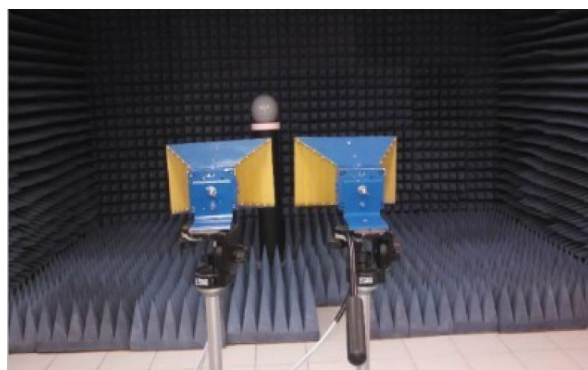
Fig. 2. Medição da refletividade do refletor de Luneberg.
