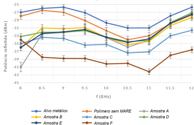
Fig. 5. Potência refletida para as amostras em função da frequência da onda EM incidente em dBm (Erro considerado de \pm 0,8 dBm).
